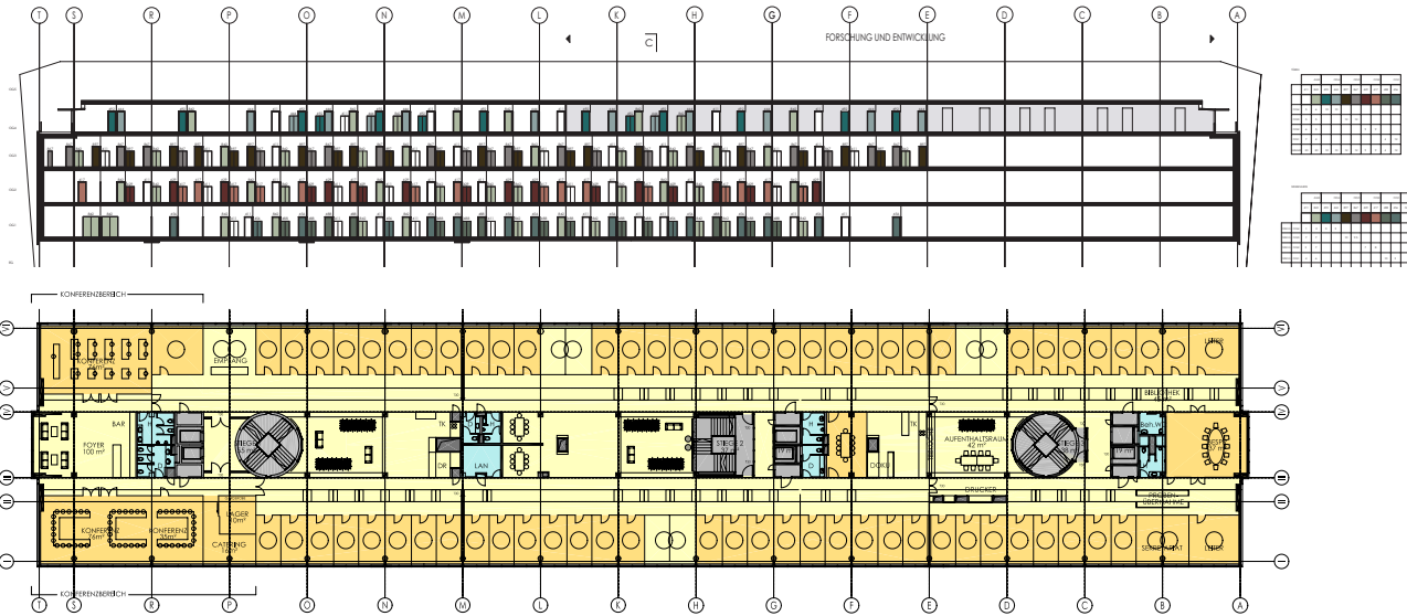
Regelgeschöß
